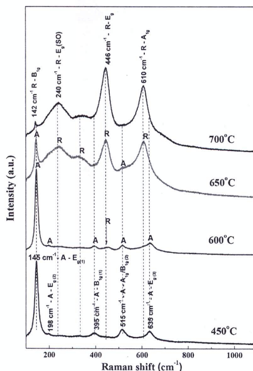
Fig. 3. Raman spectra of annealed TiO 2 nanotubes (A-anatase, R-rutile).
